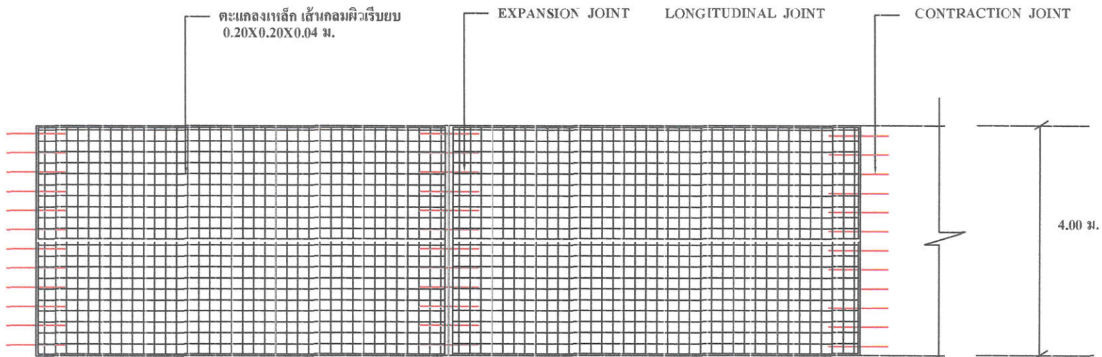
แปลนการวางตะแกรงเหล็ก
